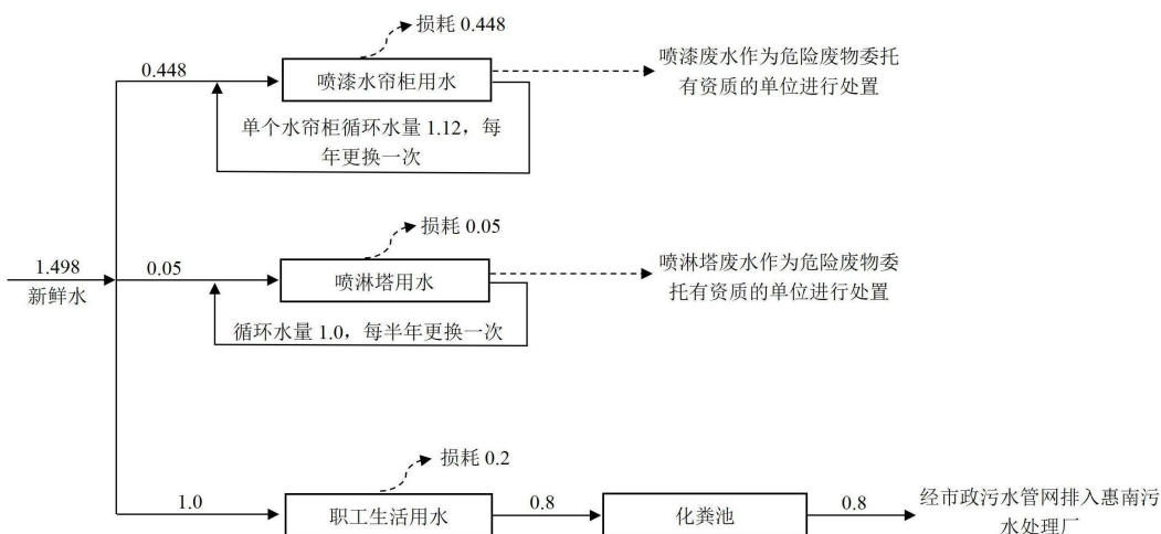
图 2-2 水平衡图 单位： \text{m}^3/\text{d}
