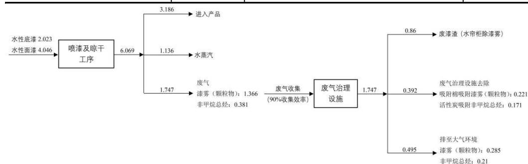
图 2-1 喷漆过程水性漆使用物料平衡 单位：t/a
